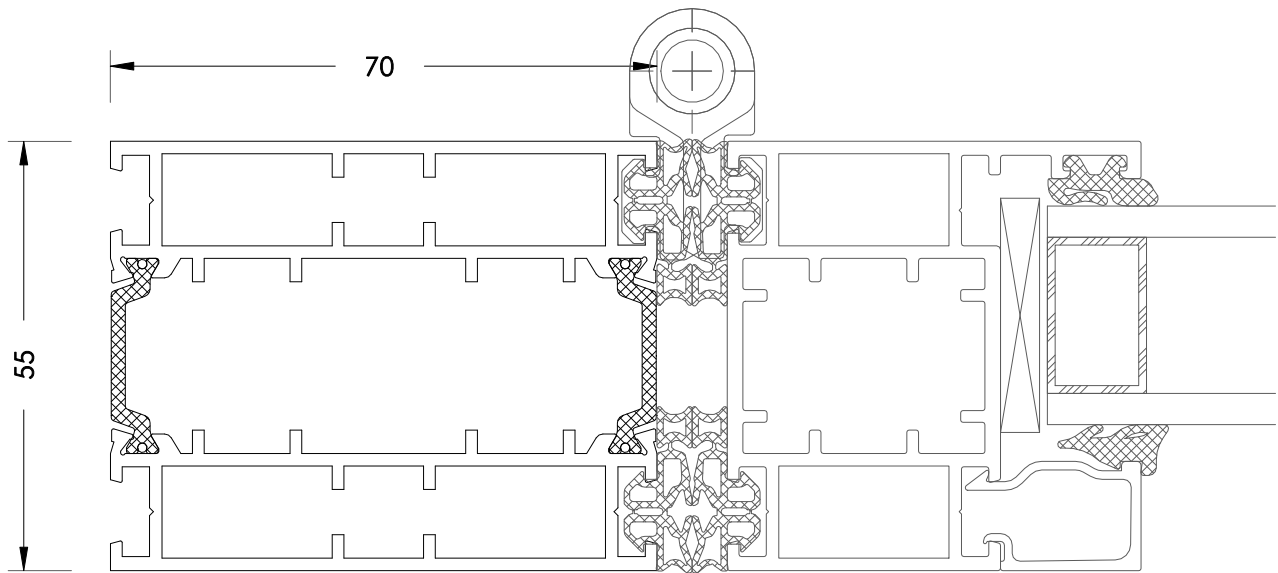
70mm Jamb
